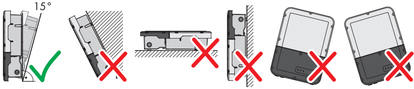
Abbildung 9: Zulässige und unzulässige Montagepositionen
