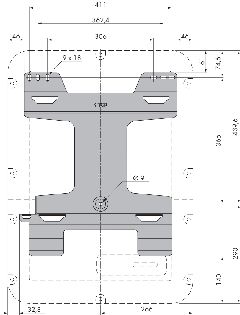
Abbildung 11: Position der Befestigungspunkte (Maßangaben in mm)
