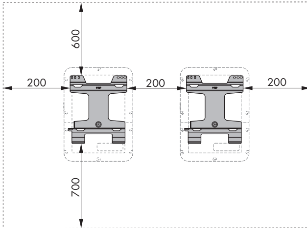
Abbildung 12: Empfohlene Abstände (Maßangaben in mm)
