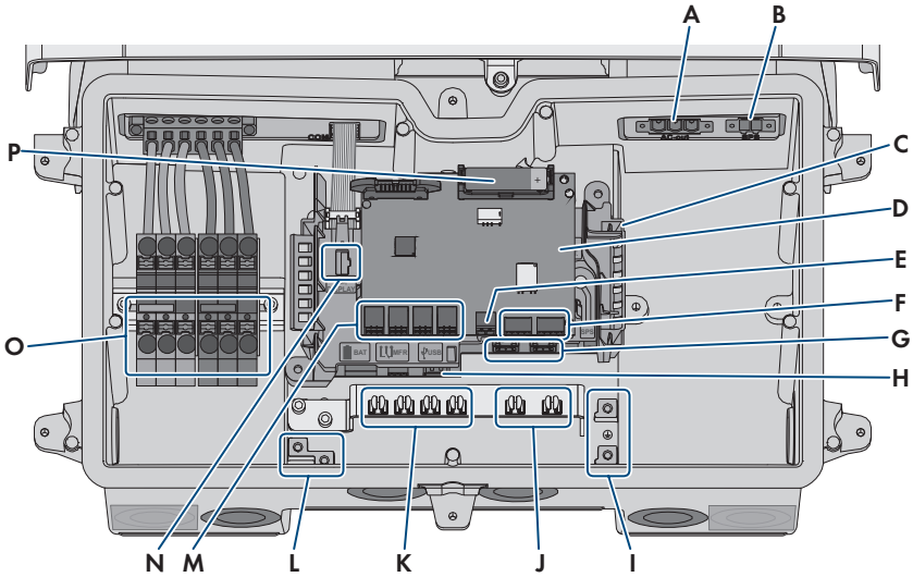
Abbildung 14: Anschlussbereiche im Inneren des Wechselrichters
